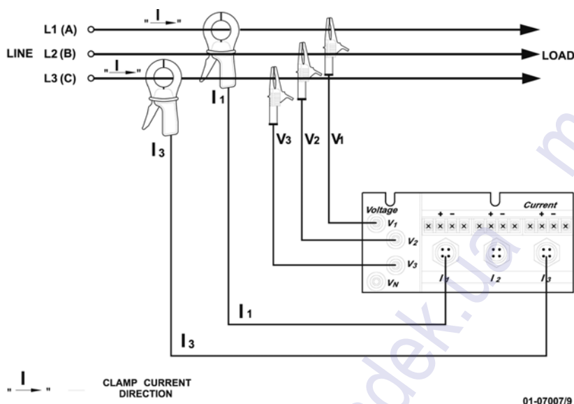
Рис.5 3-проводное прямое соединение с использованием 2 трансформаторов тока (2 элемента), Режим =3dir2.
