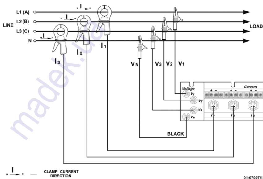
Рис.6 Четырех-проводное соединение звездой, использующее 3 трансформатора тока. Режим =4LL3 или 4Ln3
