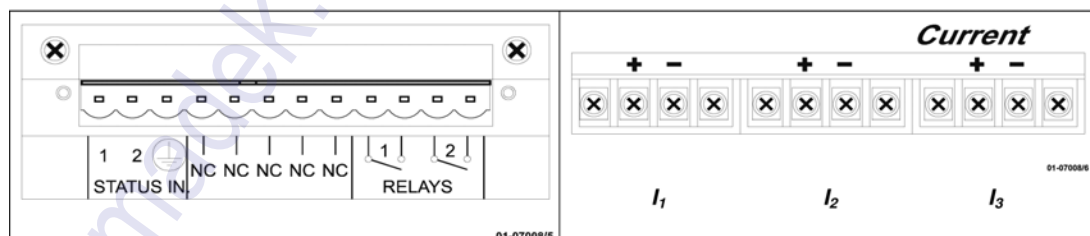
Рис.2 Общий вид клемм для подключения реле, дискретных входов и измерительных входов тока
