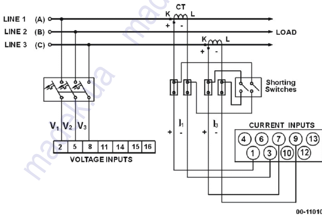
Рисунок 6 Прямое трехпроводное подключение с использованием 2 трансформаторов тока
