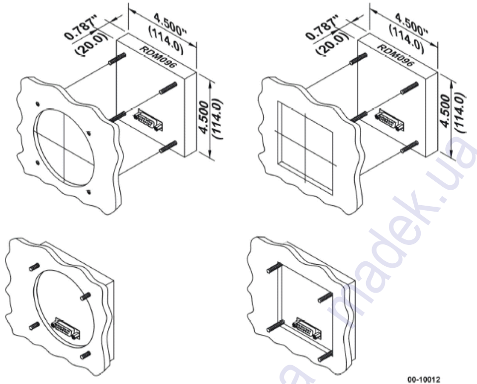
Рисунок 5 Механическая установка и размеры внешнего дисплея
